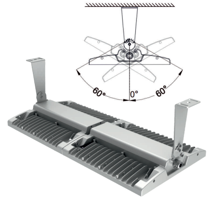
Wspornik regulowany / rotatable bracket mounting
